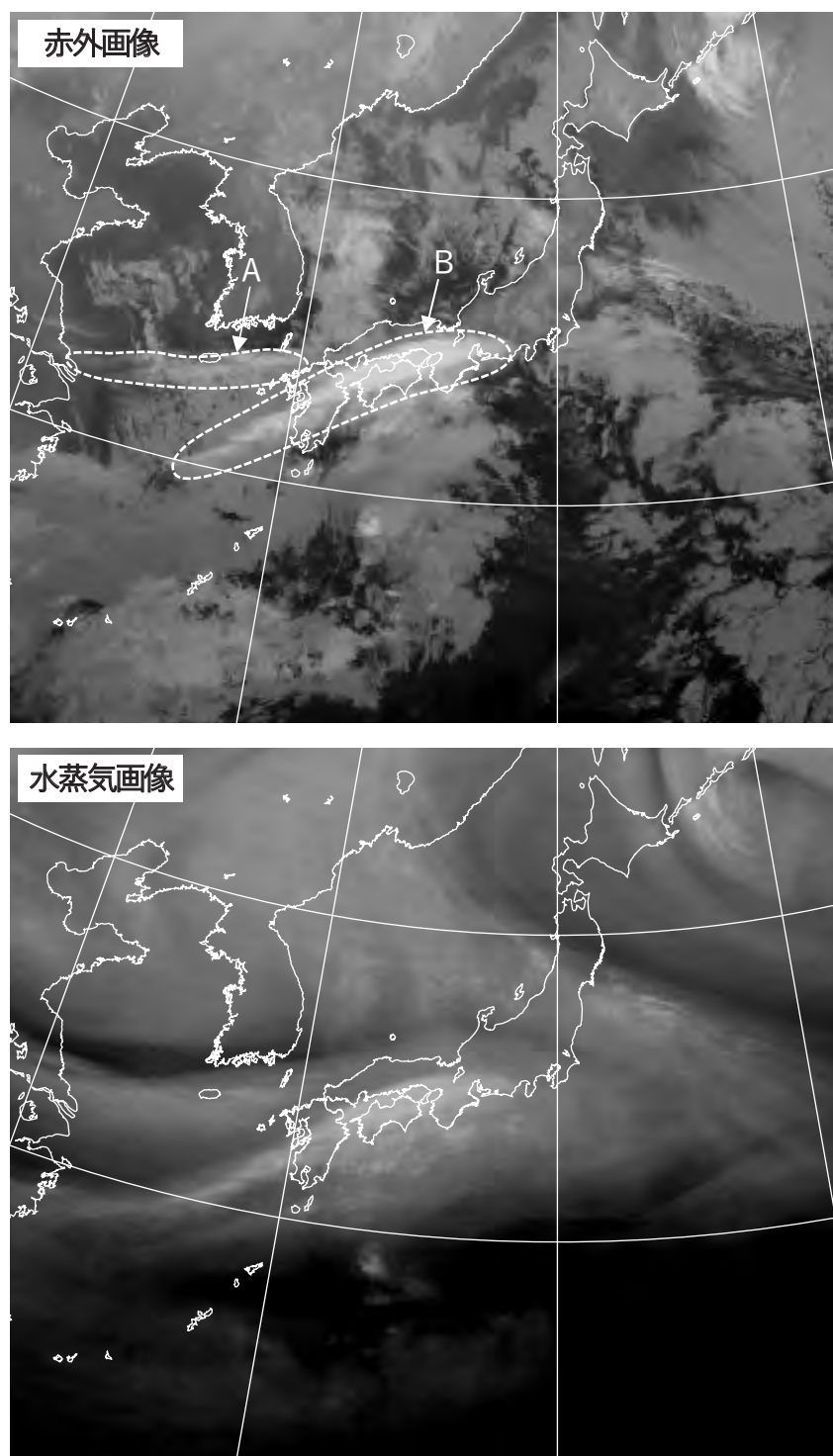
図3 気象衛星画像 赤外画像(上), 水蒸気画像(下) XX 年2月4日21時(12UTC)
