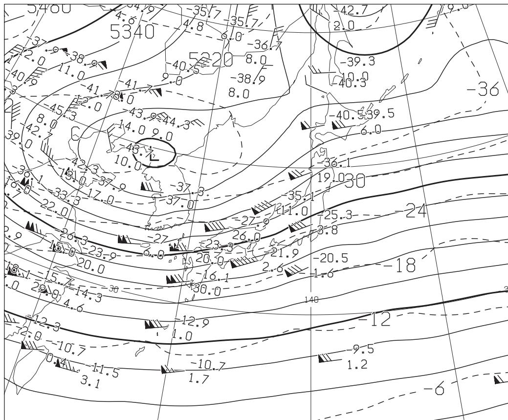
図2 500hPa 天気図
