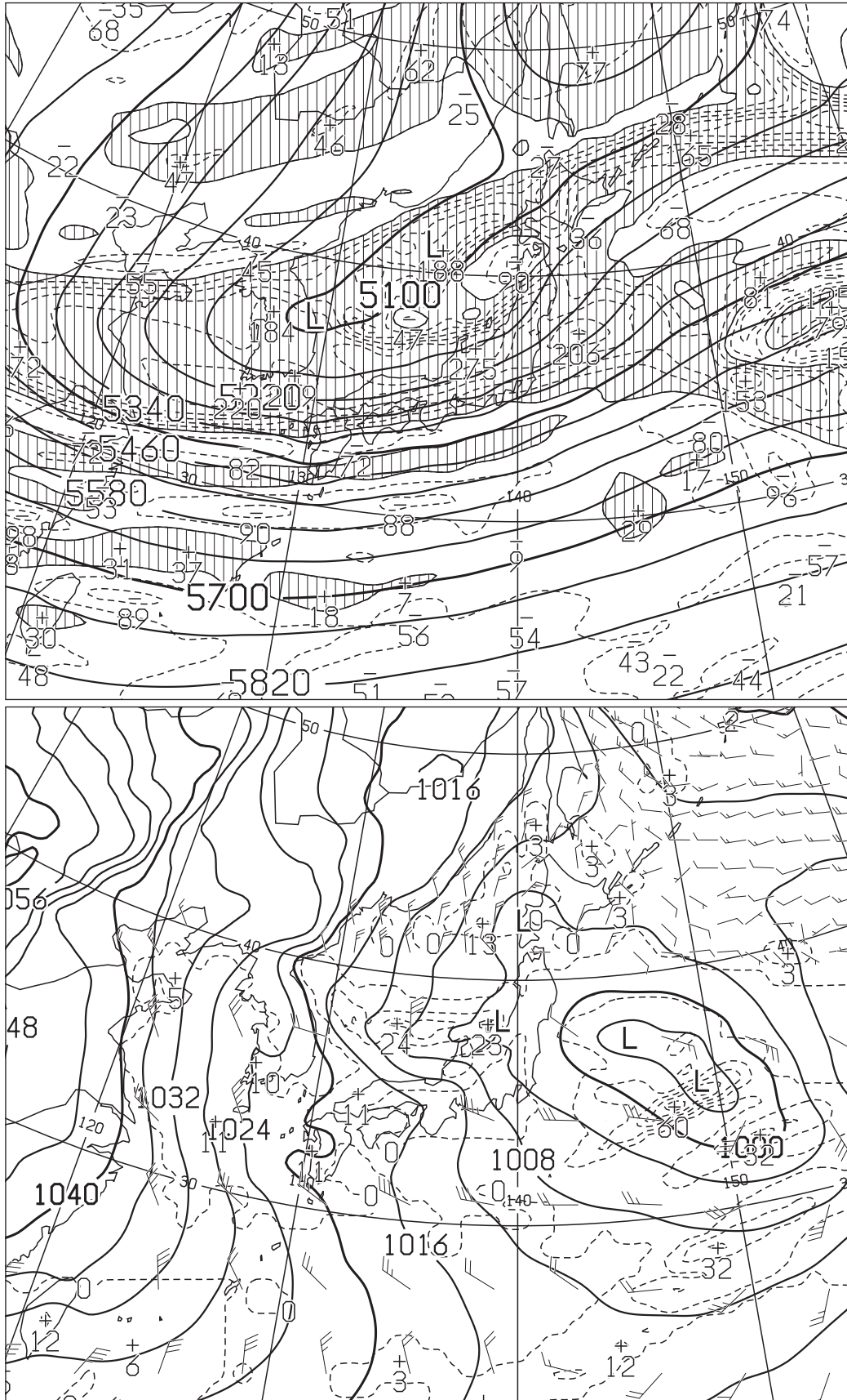
図5 500hPa 高度・渦度 12 時間予想図(上)
