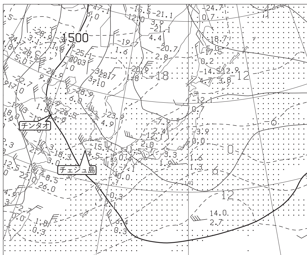
図3 850hPa 天気図
