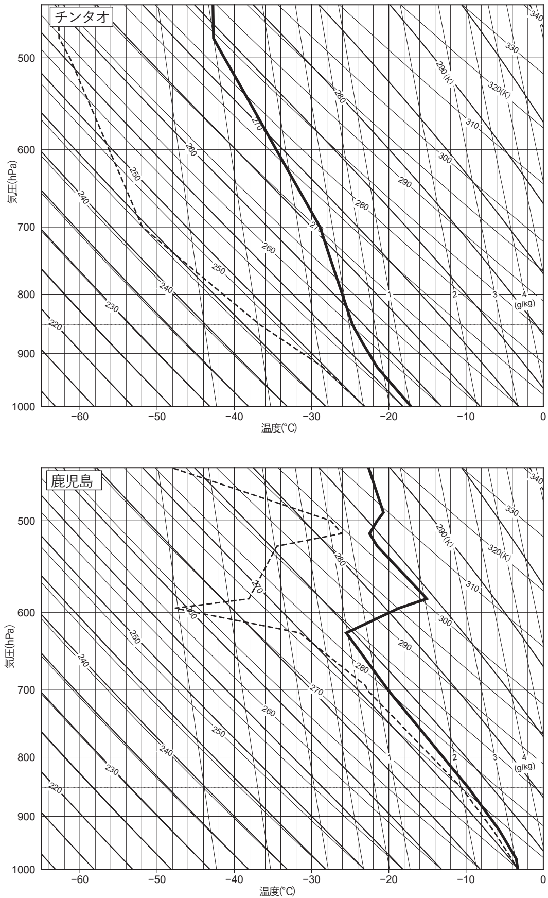
図 4 状態曲線
